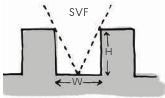
Indicateurs de forme urbaine : le facteur de vue du ciel (SVF) ou le rapport hauteur sur largeur (H/W) moyen des rues
